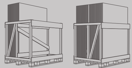
Verpackung für 20 Solarmodule
