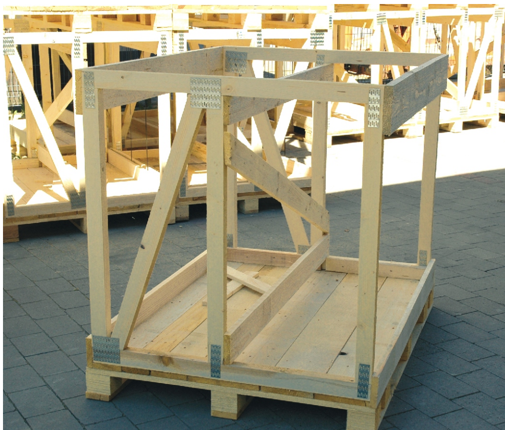
Verpackung für 20 Solarmodule
